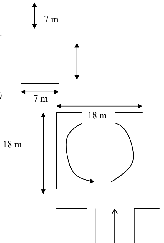
Aire de retournement (Dimensions mini., hors stationnements gênants)
